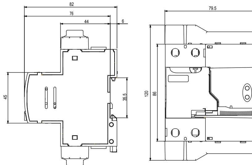
Figura 14: Dimensiones : REC 3 2 polos y REC 3C 2 polos.
