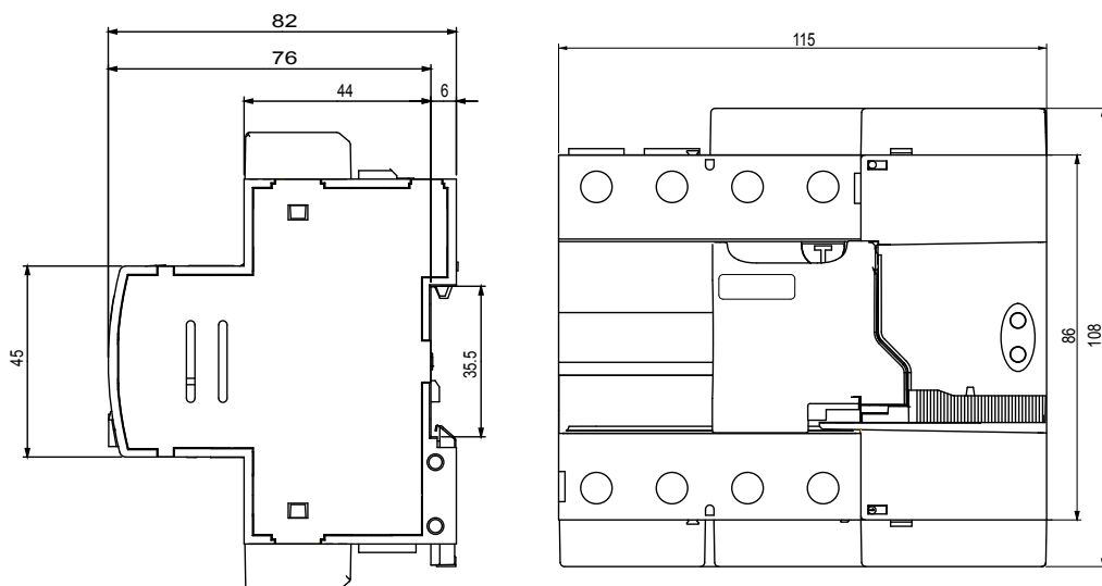
Figura 15: Dimensiones : REC 3 4 polos y REC 3C 4 polos.
